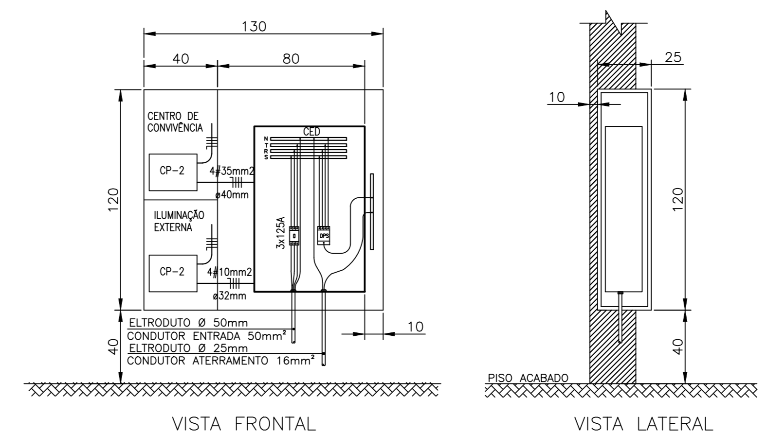
PAINEL DE MEDIDORES ESCALA: 1/20
