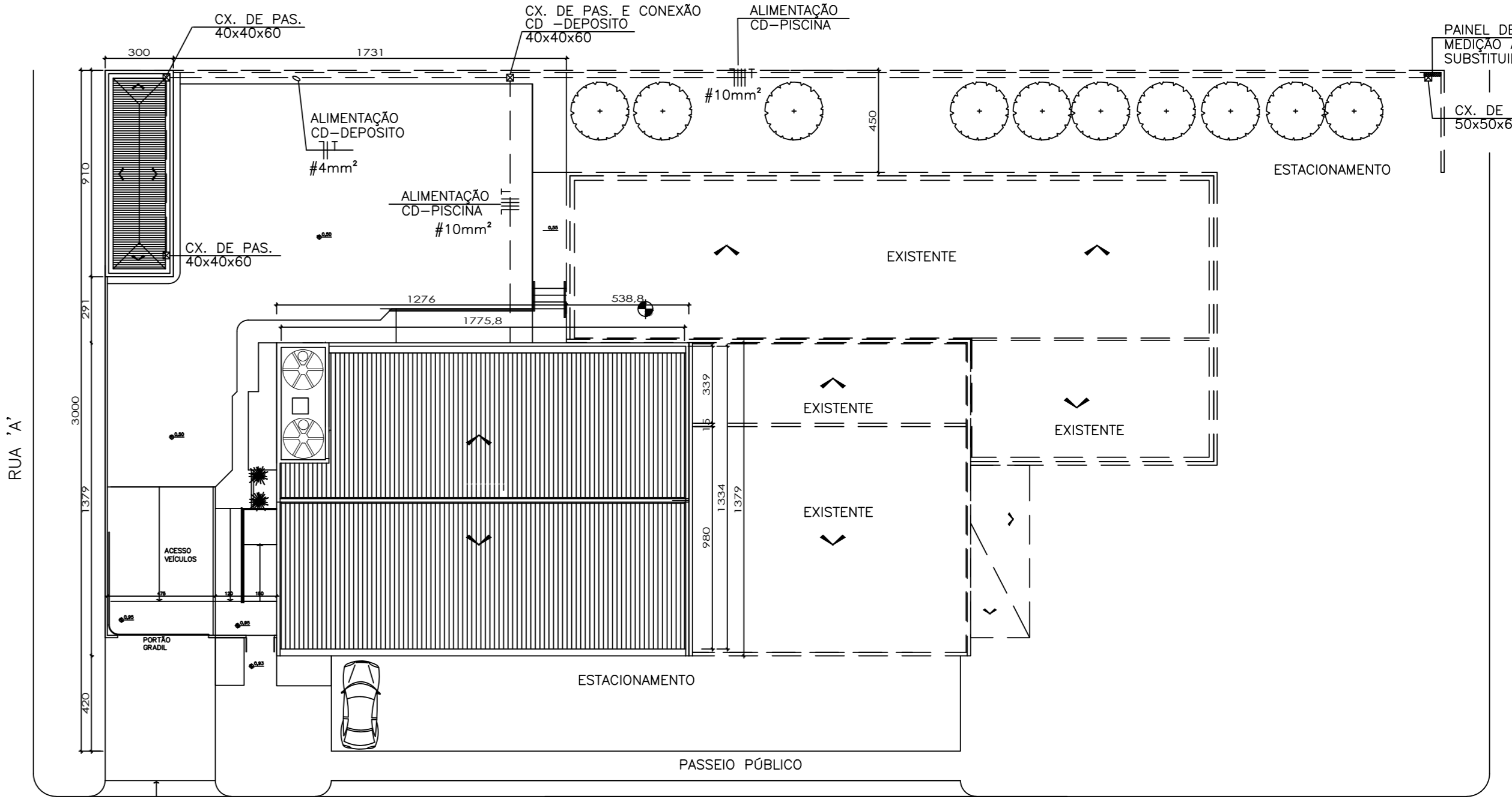
PLANTA DE LOCALIZAÇÃO ESCALA: 1/200
