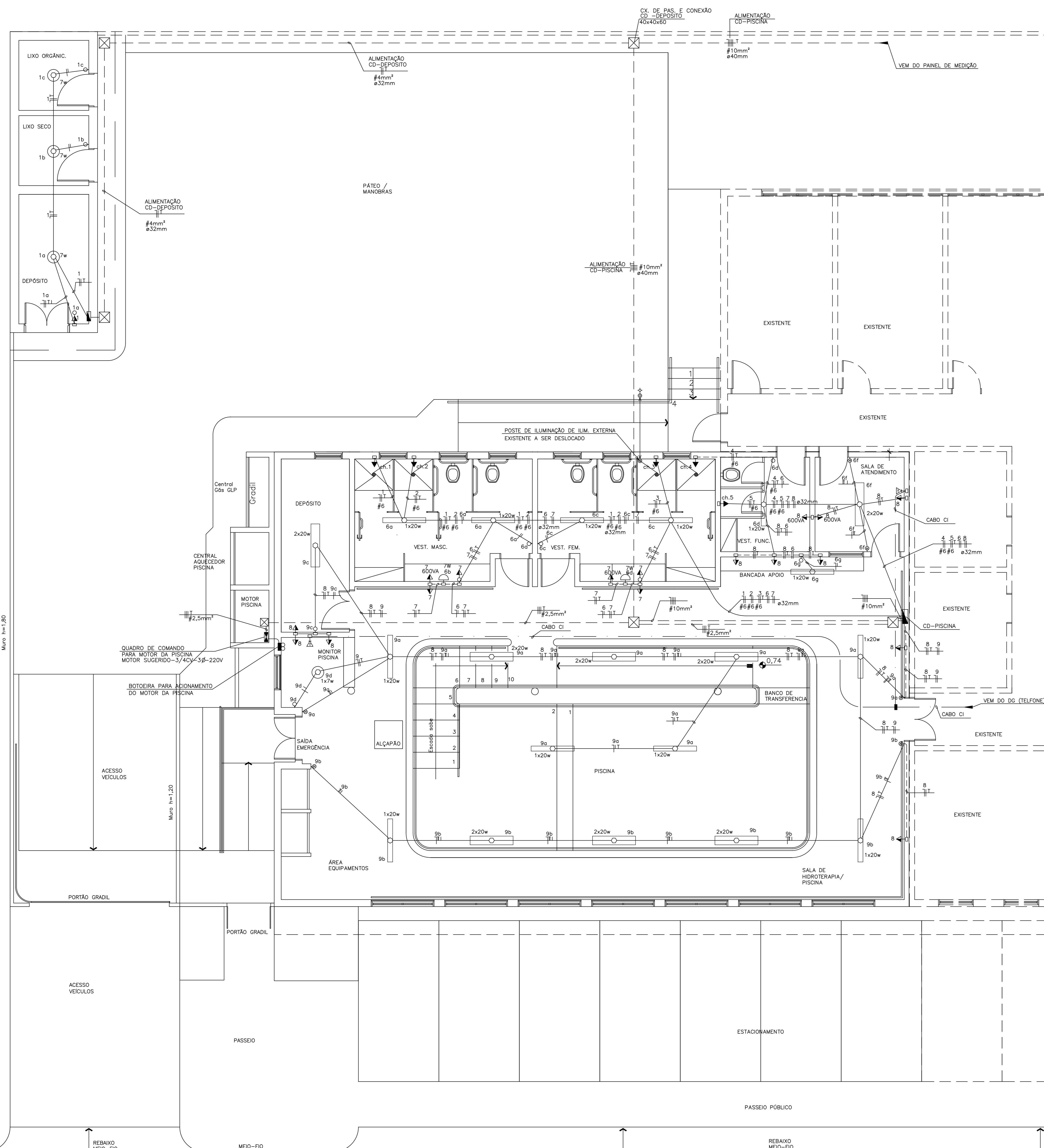
PLANTA BAIXA ESCALA: 1/50
